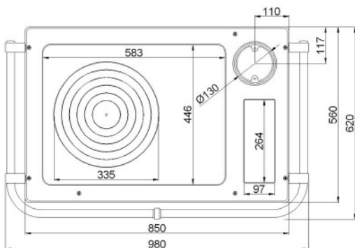
Bild 2 (Draufsicht)
