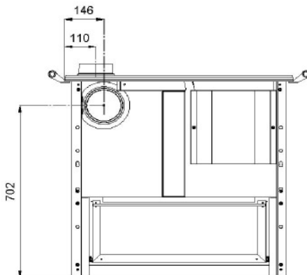
Bild 3 (Rückansicht)
