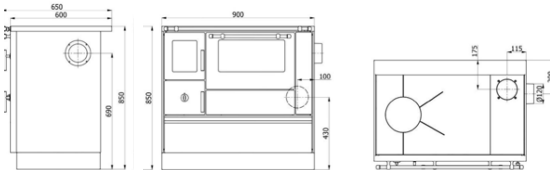
Holzherd K 76F 90, Schwarz mit Ceranplatte
