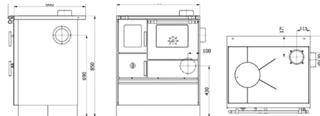
Style 70F, Schwarz mit Stahlplatte
